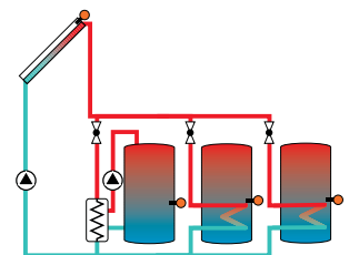
Solarsystem mit 3 Speichern (Pufferspeicher mit ext. Wärmetauscher) 1 Kollektor / 3 Speicher
