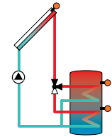
Solarsystem mit Speicherschichtladung 1 Kollektor / 1 Speicher
