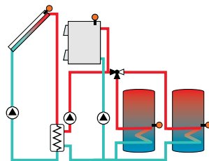
Solarsystem mit zus. Wärmequelle (Feststoffkessel) 1 Kollektor / 2 Speicher
