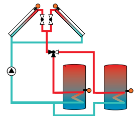
Solarsystem mit Ost- / Westdach 2 Kollektoren / 2 Speicher
