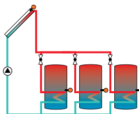
Solarsystem mit 3 Speichern 1 Kollektor / 3 Speicher
