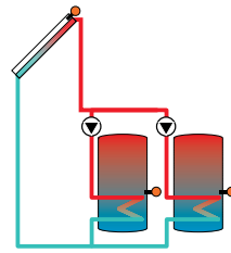
Solarsystem mit 2 Speichern (Pumpensteuerung) 1 Kollektor / 2 Speicher
