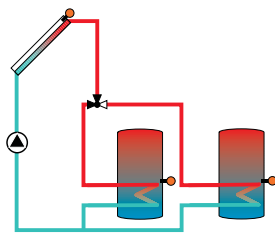
Solarsystem mit 2 Speichern (Ventilsteuerung) 1 Kollektor / 2 Speicher
