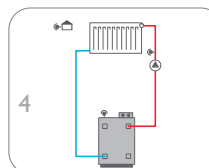
Un circuito de calefacción sin mezcla y con calentamiento auxiliar
