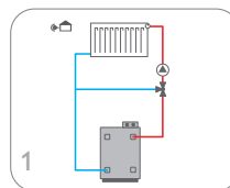
Un circuito de calefacción con mezcla
