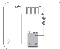
Un circuito de calefacción con mezcla y calentamiento auxiliar
