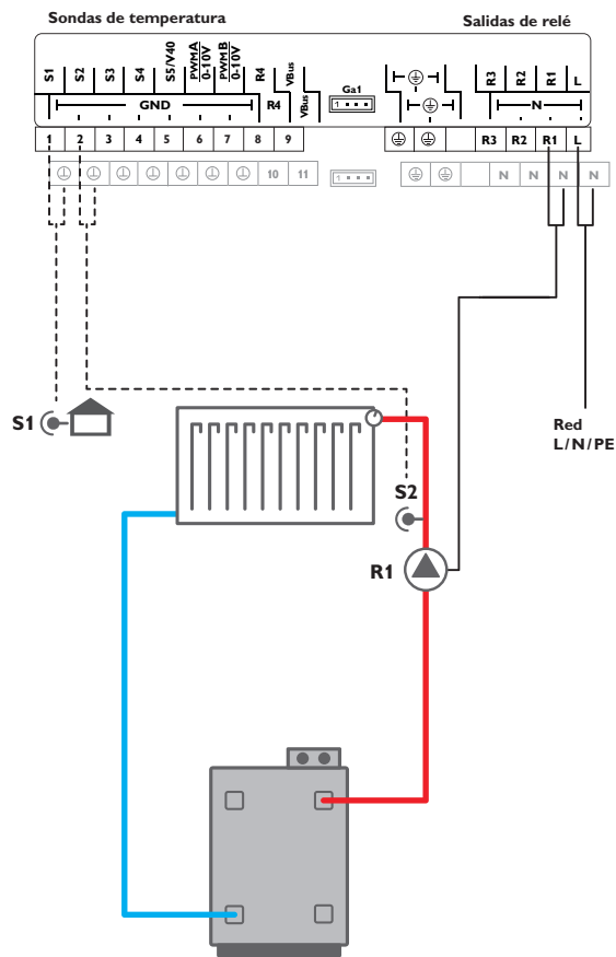
Esquema 3: un circuito de calefacción sin mezcla
