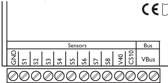
Masse-Sammelklemmenblock
