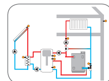
Solarsystem mit Kombispeicher, externem Wärmetauscher, witterungsgeführtem Heizkreis, Rücklaufanhebung und Nachheizung
