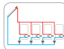
Solarsystem mit 4 Speichern Pumpensteuerung
