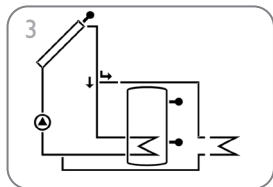
Sistema de energía solar con evacuación del calor excedente (página 17)
