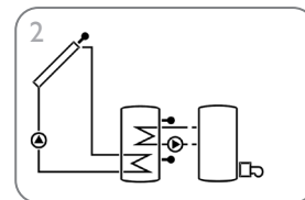
Sistema de energía solar con calentamiento auxiliar (página 12)
