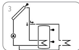
Impianto solare standard con asportazione del calore in eccesso (pagina 17)
