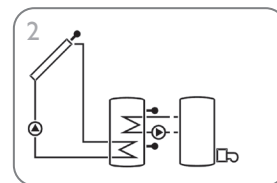
Impianto solare con riscaldamento integrativo (pagina 12)
