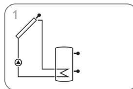
Impianto solare standard (pagina 9)
