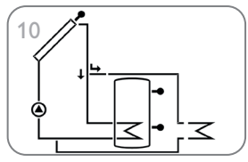
Impianto solare standard con asportazione del calore in eccesso (pagina 45)
