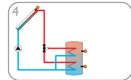
Système de chauffage solaire avec 1 réservoir et 1 vanne à 3 voies pour la charge stratifiée du réservoir (page 12)
