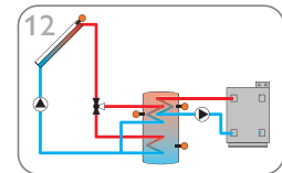
Système de chauffage solaire avec 1 réservoir stratifié et chauffage d'appoint (page 20)
