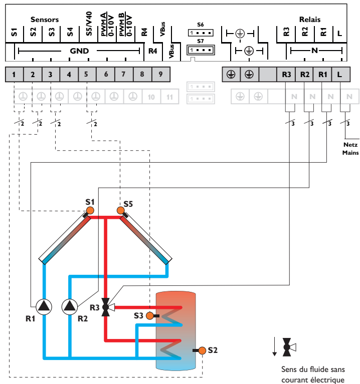
Variante hydraulique 1
