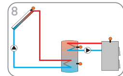
Système de chauffage solaire avec 1 réservoir et 1 chaudière à combustible solide (page 16)
