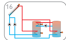
Système de chauffage solaire avec 2 réservoirs, logique de pompe et échange de chaleur (page 24)
