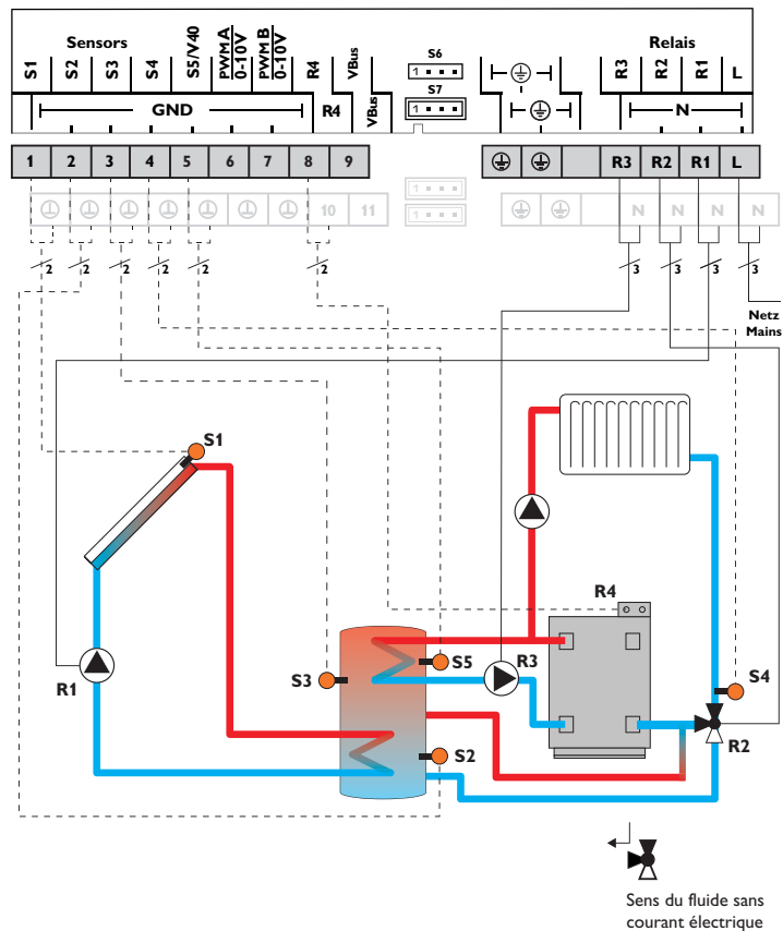
Variante hydraulique 1
