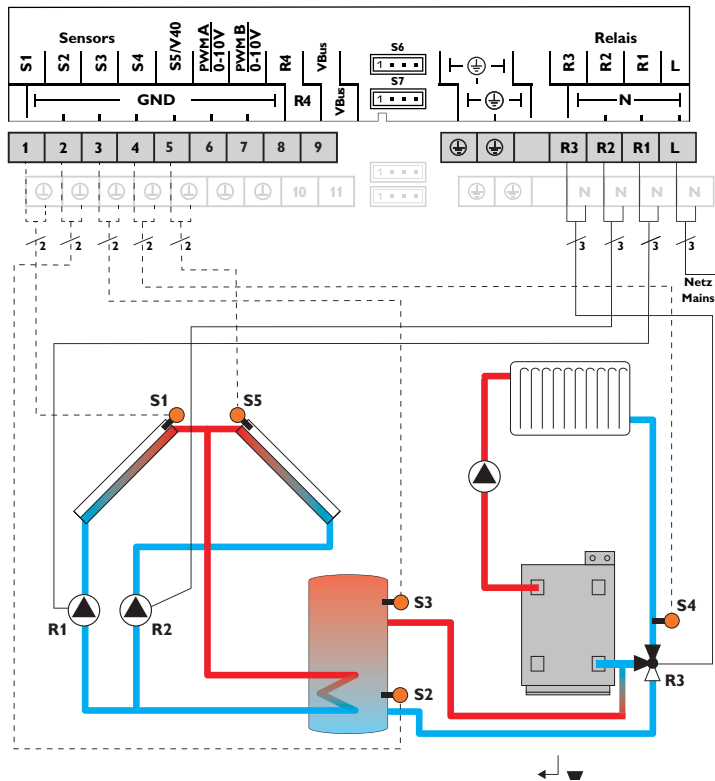
Variante hydraulique 1
