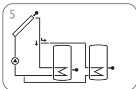
Sistema solar de 2 acumuladores com lógica de válvula (pág. 25)
