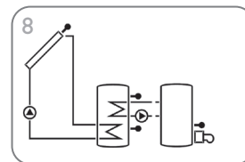
Zonnestelsysteem met naverwarming door vaste-brandstofketel (pagina 36)
