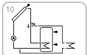
Standaardzonnestelsysteem met restwarmteafvoer (pagina 45)
