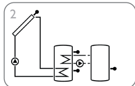
Zonnestelsysteem met warmtewisseling (pagina 13)
