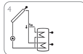
Zonnestelsysteem met gelaagde buffering (pagina 24)
