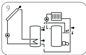
Zonnestelsysteem met verwarmingscircuit-retourverhoging (pagina 42)
