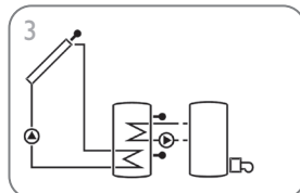
Zonnestelsysteem met naverwarming (pagina 19)
