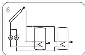
Zonnestelsysteem met 2 boilers met pomplogica (pagina 30)
