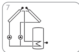
Zonnestelsysteem met 2 collectoren en 1 boiler (pagina 33)
