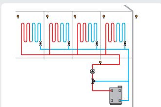
1 circuit de chauffage mélangé avec 4 zones
