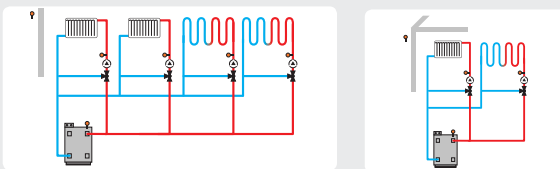
4 circuits de chauffage mélangés avec chauffage d'appoint (demande) 2 circuits de chauffage mélangés avec chauffage d'appoint (demande)
