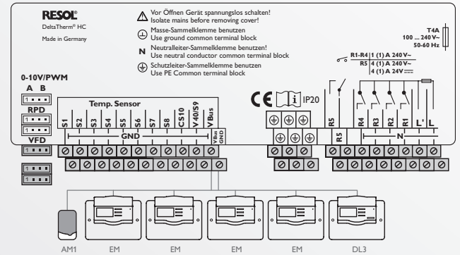
1 circuit de chauffage mélangé avec source de chaleur externe (p. ex. chauffage urbain) 1 circuit de chauffage mélangé avec chauffage d'appoint (demande) 1 circuit de chauffage mélangé avec chauffage d'appoint (demande) et pompe de charge chaudière) 1 circuit de chauffage mélangé avec source de chaleur externe (p. ex. chauffage urbain)
