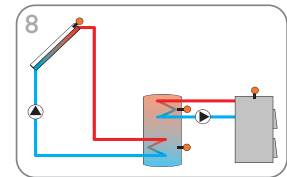
Système de chauffage solaire avec 1 réservoir et 1 chaudière à combustible solide (page 17)
