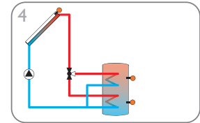
Système de chauffage solaire avec 1 réservoir et 1 vanne à 3 voies pour la charge stratifiée du réservoir (page 13)
