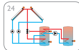
24 Sistema de energía solar con captadores este/oeste e intercambio de calor (página 33)
