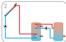
Sistema solar con 2 acumuladores e intercambio de calor (página 11)
