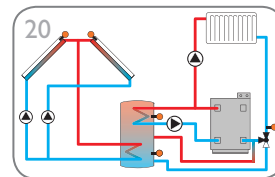
20 Sistema de energía solar con captadores este/oeste, aumento de temperatura de retorno y calentamiento auxiliar termostático (página 29)
