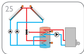
25 Sistema de energía solar con captadores este/oeste y calentamiento auxiliar (página 34)
