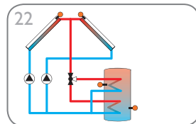
22 Sistema de energía solar con captadores este/oeste y 1 acumulador estratificado (página 31)
