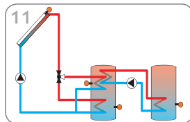
Sistema de energía solar con 1 acumulador estratificado e intercambio de calor (página 20)
