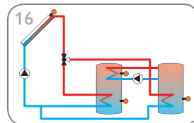
Sistema de energía solar con 1 acumulador estratificado e intercambio de calor (página 25)
