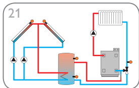
21 Sistema de energía solar con captadores este/oeste y aumento de temperatura de retorno (página 30)
