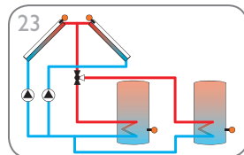
23 Sistema de energía solar con captadores este/oeste, 2 acumuladores y lógica de válvula (página 32)
