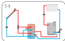
Sistema de energía solar con 1 acumulador estratificado y aumento de temperatura de retorno (página 23)
