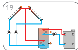
19 Sistema de energía solar con captadores este/oeste y calentamiento auxiliar (página 28)
