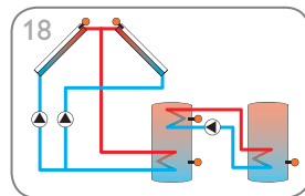
18 Sistema de energía solar con captadores este/oeste, 2 acumuladores, lógica de bomba e intercambio de calor (página 27)
