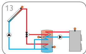
Sistema de energía solar con 1 acumulador estratificado y 1 caldera de biomasa (página 22)
