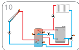
Sistema de energía solar con 1 acumulador, aumento de temperatura de retorno y calentamiento auxiliar (página 19)
