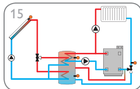
Sistema de energía solar con 1 acumulador estratificado, aumento de temperatura de retorno y calentamiento auxiliar (página 24)
