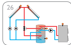
26 Sistema de energía solar con captadores este/oeste y caldera de biomasa (página 35)
