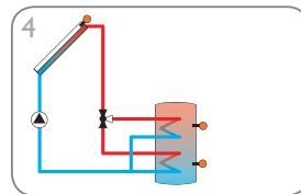
Sistema de energía solar con 1 acumulador y 1 válvula de 3 vías para la carga estratificada del acumulador (página 12)
