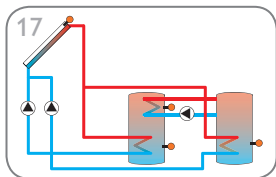
17 Sistema de energía solar con 2 acumuladores, lógica de válvula e intercambio de calor (página 26)
