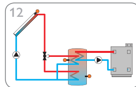
Sistema de energía solar con 1 acumulador estratificado y calentamiento auxiliar (página 21)
