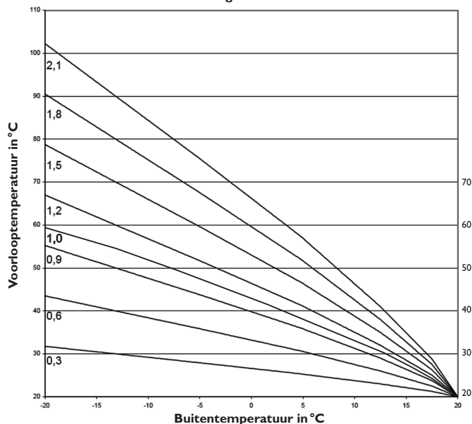
Verwarmingskarakteristieken
