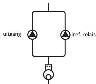
Voorbeeldschema voor twelingpompen in de zonne-energieaanvoer met voorgeschakeld volumemete gedeelte
