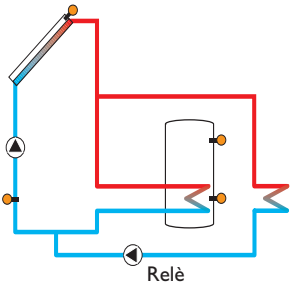
Variante pompa
