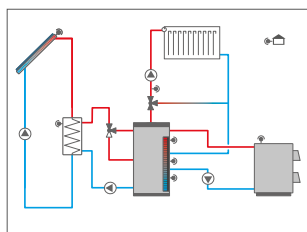
Sistema de energía solar con 1 intercambiador de calor externo, 1 acumulador estratificado y calentamiento auxiliar mediante caldera de biomasa
