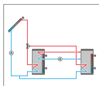
Sistema de energía solar con 2 acumuladores y función de intercambio térmico por válvula
