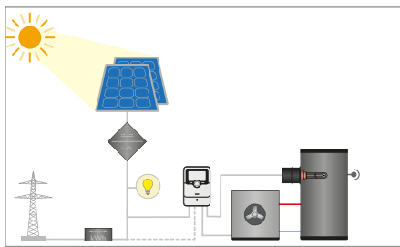
Control de una resistencia eléctrica de calentamiento* y bomba de calor
