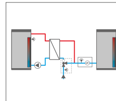
Precalentamiento ACS
