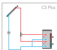
Sistema solar con 1 acumulador estratificado
