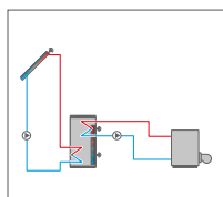
Sistema de energía solar con 1 acumulador y calentamiento auxiliar
