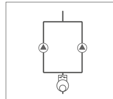
Bomba paralela
