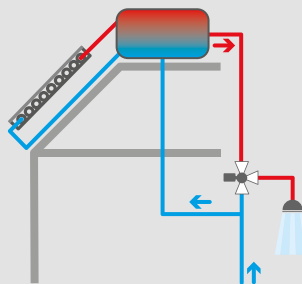
Sistema termosifón
