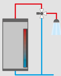
Sistema solar de producción ACS
