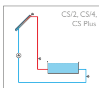
Sistema de energía solar con piscina*
