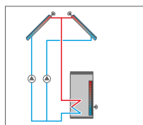
Sistema solar con 1 acumulador y captadores este/oeste
