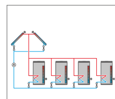
Sistema de energía solar con 4 acumuladores, captadores este/oeste, funcionamiento por válvula
