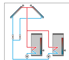
Sistema de energía solar con 2 acumuladores, captadores este/oeste, funcionamiento por válvula/bomba
