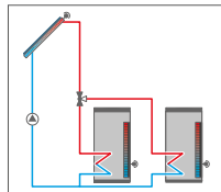
Sistema solar con 2 acumuladores, funcionamiento por válvula
