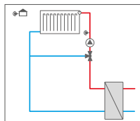
1 circuito de calefacción mezclado con calentamiento auxiliar (p.ej. calefacción urbana)
