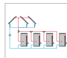
Sistema de energía solar con 3 campos de captadores, 4 acumuladores, funcionamiento por válvula y válvulas de inversión
