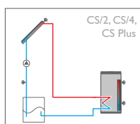
Sistema de energía solar drainback*
