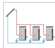
Sistema de energía solar con 3 acumuladores, funcionamiento por bomba
