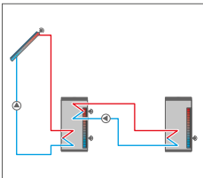
Intercambio térmico
