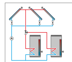
Sistema de energía solar con 3 campos de captadores, 2 acumuladores, funcionamiento por válvula y válvulas de inversión
