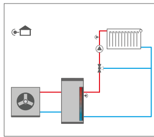
1 circuito de calefacción mixto con 1 acumulador y bomba de calor (demanda)
