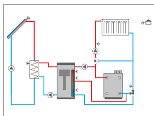
Sistema de energía solar con 1 acumulador combinado, 1 intercambiador de calor externo, 1 bomba de circulación, 1 intercambiador de calor y 1 circuito de calefacción controlado en función de la temperatura exterior; aumento de temperatura del retorno y calentamiento auxiliar
