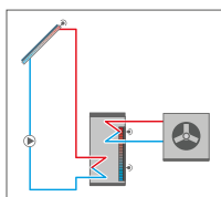
Sistema de energía solar con 1 acumulador y calentamiento auxiliar mediante bomba de calor
