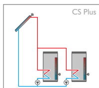
Sistema solar con 2 acumuladores, funcionamiento por bomba
