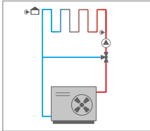
1 circuito de calefacción mixto para calefacción y refrigeración
