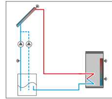
Sistema drainback con bomba booster
