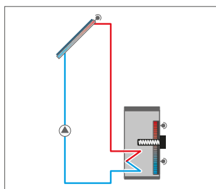
Sistema solar con calentamiento auxiliar eléctrico (esquema simplificado en la pantalla del regulador)
