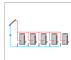
Sistema de energía solar con 5 acumuladores, funcionamiento por válvula
