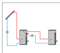
Sistema de energía solar con 1 acumulador y 1 función de intercambio térmico
