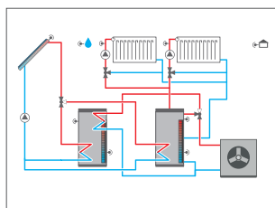
Système de chauffage solaire à 2 réservoirs et 2 circuits de chauffage dépendants des conditions climatiques extérieures pour le chauffage ou le refroidissement à travers une pompe à chaleur et calcul du point de rosée à l'aide de la sonde d'humidité FRH(d)
