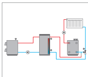
Chaudière à combustible solide avec augmentation de la température de retour du circuit de chauffage
