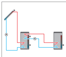
Fonction échange de chaleur
