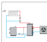
1 circuit de chauffage mélangé avec chaudière à combustible solide et chauffage d'appoint à travers une pompe à chaleur (demande)
