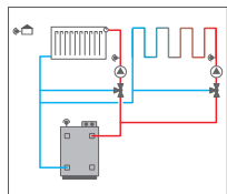
2 circuits de chauffage mélangés avec chauffage d'appoint (demande)
