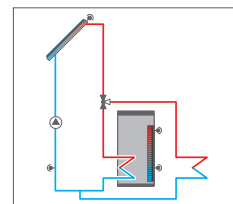
Evacuation de l'excès de chaleur
