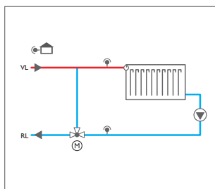
Système de base avec vanne mélangeuse
