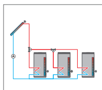
Système de chauffage solaire à 3 réservoirs, commande vanne à 3 voies
