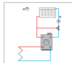
Refroidissement à travers le circuit de chauffage (p. ex. avec une pompe à chaleur)
