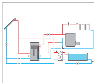
Système de chauffage solaire avec 1 réservoir multifonctionnel et piscine, chauffage d'appoint, chauffage du circuit et augmentation de température de retour
