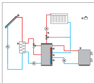
Système avec échangeur de chaleur externe, réservoir stratifié et chauffage d'appoint à travers chaudière combustible solide
