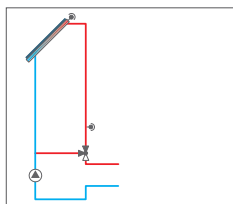
Logique de vanne bypass
