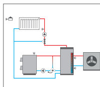
1 circuit de chauffage mélangé avec chaudière à combustible solide et chauffage d'appoint à travers une pompe à chaleur (demande)
