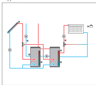
Système à 2 réservoirs, commande pompe circulation, chaudière combustible solide et circuit de chauffage dépendant des conditions climatiques
