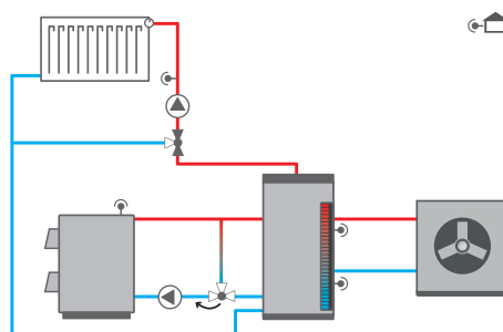
DeltaTherm® HC Plus et DeltaSol® BX Plus
