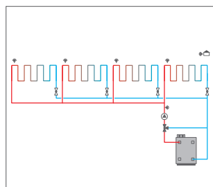
1 circuit de chauffage mélangé avec 4 zones
