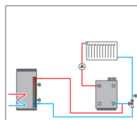
Augmentation de température retour dans le circuit de chauffage
