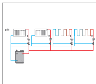
4 circuits de chauffage mélangés avec chauffage d'appoint (demande)
