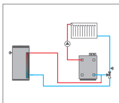
Augmentation de la température du retour
