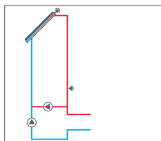
Logique de pompe bypass
