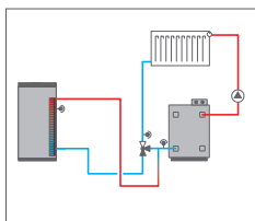
Maintien de la température retour
