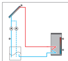
Système drainback avec pompe booster
