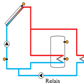
Variante Pumpe
