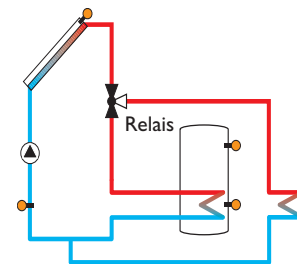
Variante Ventil
