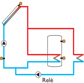
Variante pompa
