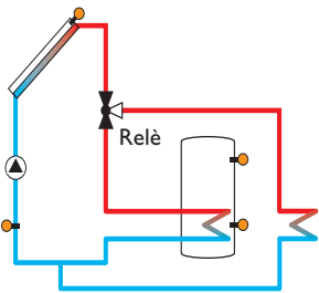
Variante valvola
