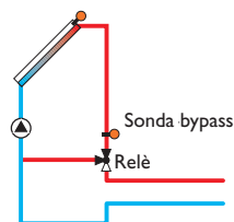
Variante valvola:
