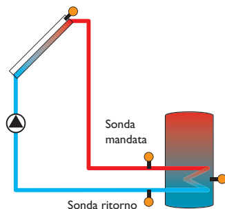
Esempio di posizionamento delle sonda mandata e ritorno
