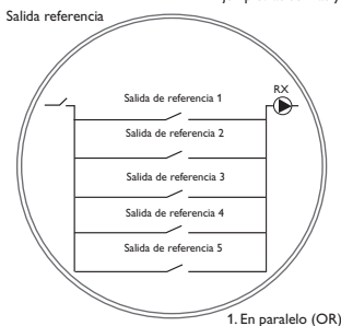
1. En paralelo (OR)
