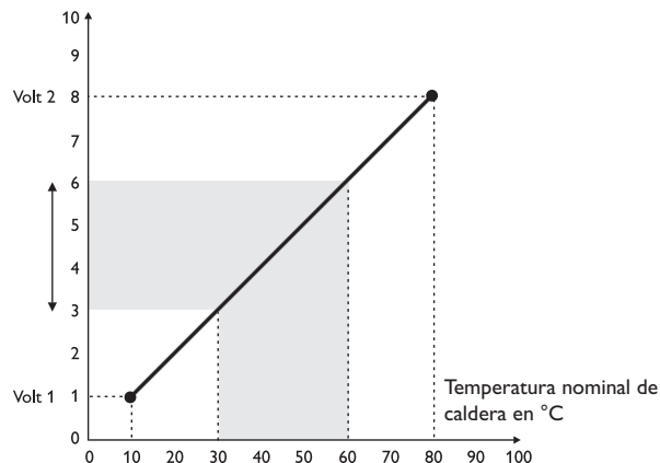
Señal de tensión en V
