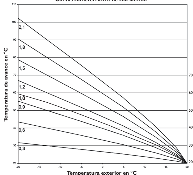
Curvas características de calefacción
