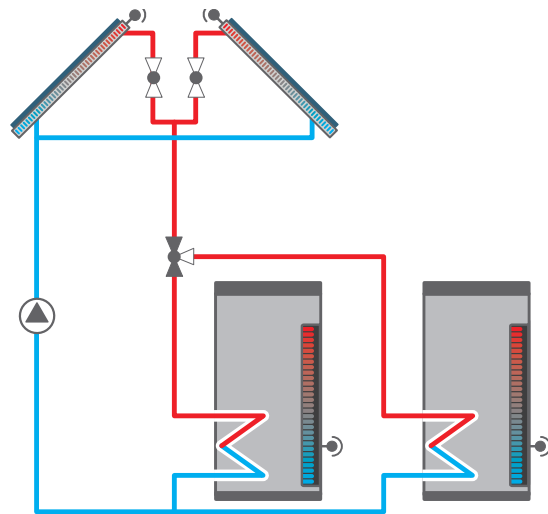
Solarsystem mit 2 Kollektoren, 2 Speichern und 3-Wege-Ventil zur Umschaltung zwischen den Speichern.
