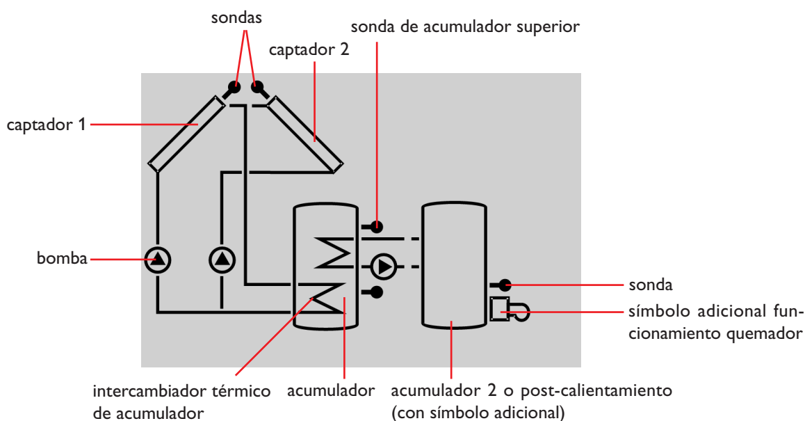
captadores con sonda de captador
