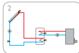
Impianto solare con riscaldamento integrativo (pagina 10)
