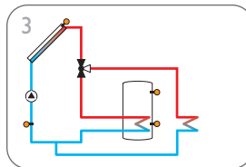
Impianto solare standard con asportazione del calore in eccesso (pagina 14)
