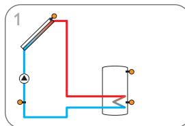
Impianto solare standard (pagina 8)
